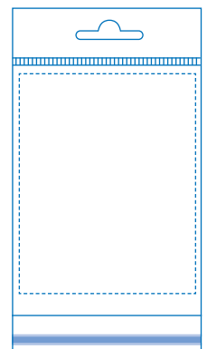
Headerbeutel mit Euroloch, 2 bzw. 3 Kammern innen, Klappe, Adhäsionsverschluss und Öffnung unten
