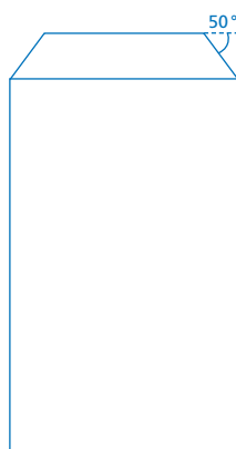
Klappenbeutel mit angeschrägten Ecken
